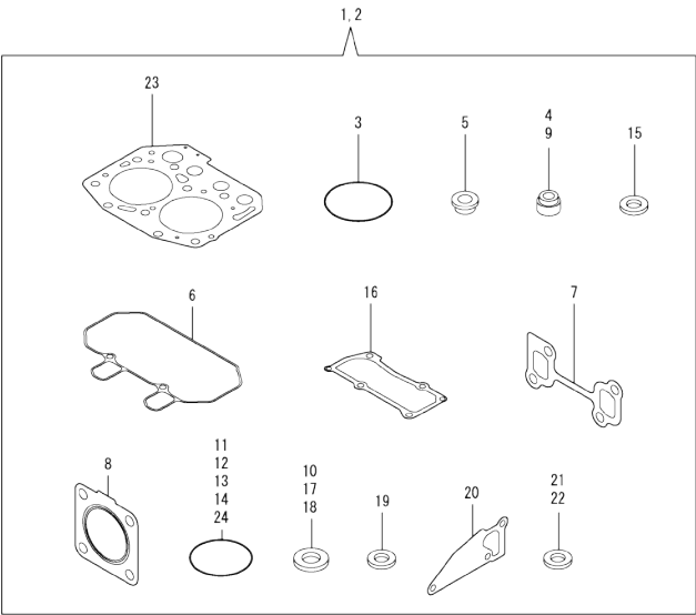
Fig.16. GASKET SET
