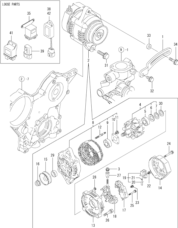
Fig.15. GENERATOR
